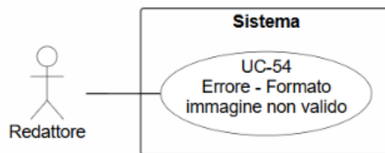
Figura 83: Diagramma del caso d'uso UC-54: Errore per formato immagine non valido
