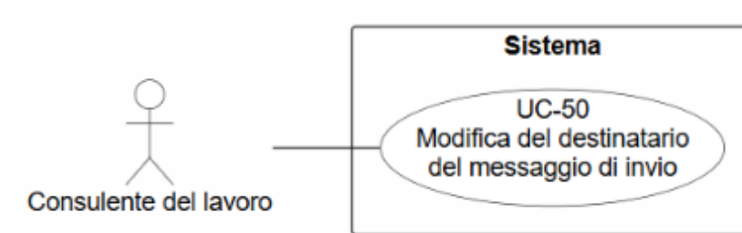
Figura 74: Diagramma del caso d'uso UC-50: Modifica del destinatario del messaggio di invio
